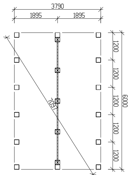
Plintritning
