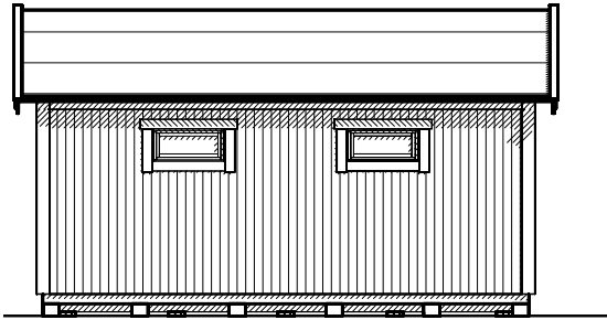
Långsida
