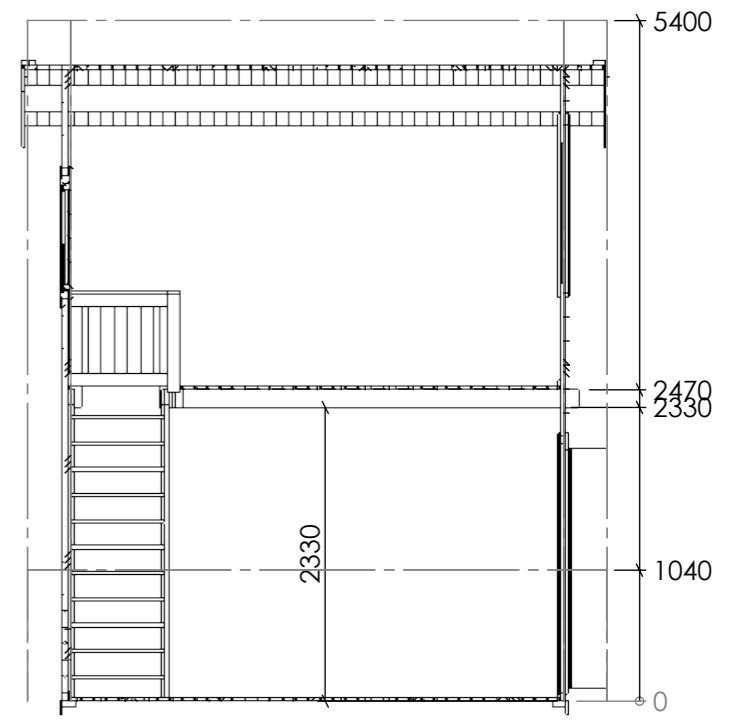
C-C 1
