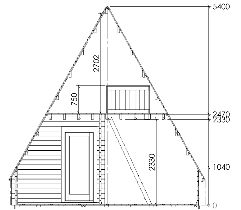
C-C 2
