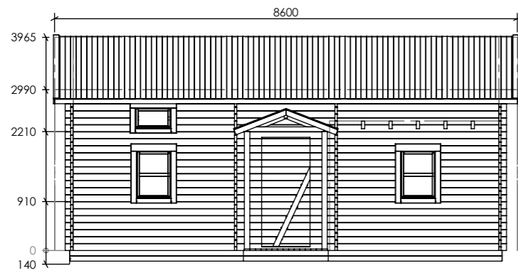
Facade A-B
