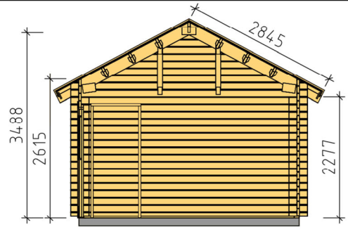
SEKTION A-A
